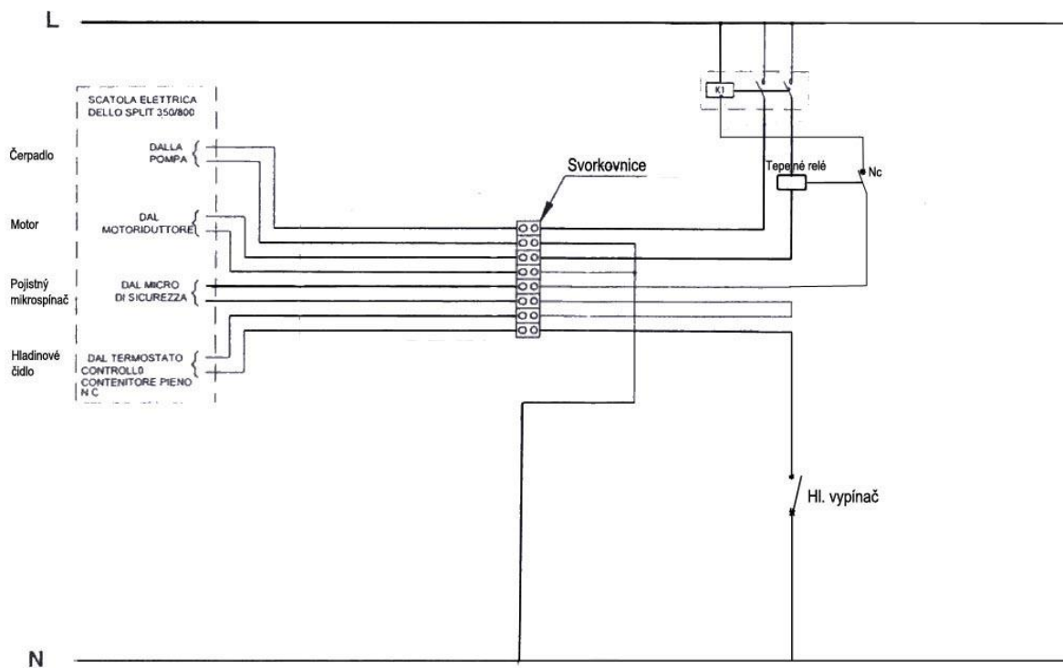
SCHÉMA ELEKTRICKÉHO ZAPOJENÍ MODELU SPLIT 1750
